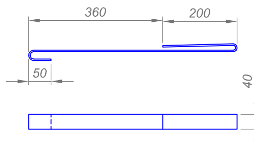
Деталь 6
