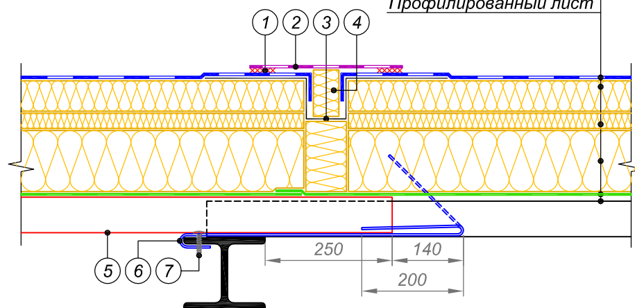
Деталь 3
